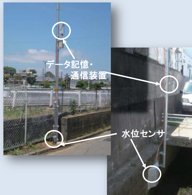
▲ 水位センサの設置状況
